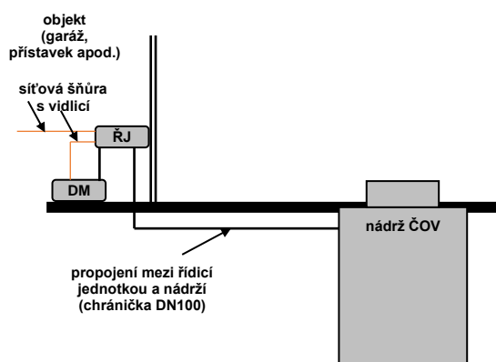
umístění dmyhadla v objektu
