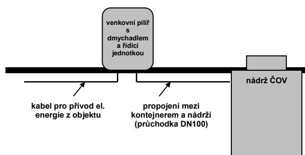
umístění dmyhadla v piliři u nádrže
